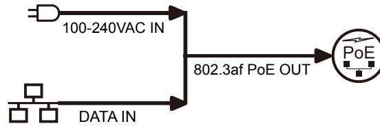
GigE 802.3af PoE Injector TP-POE-48GD
